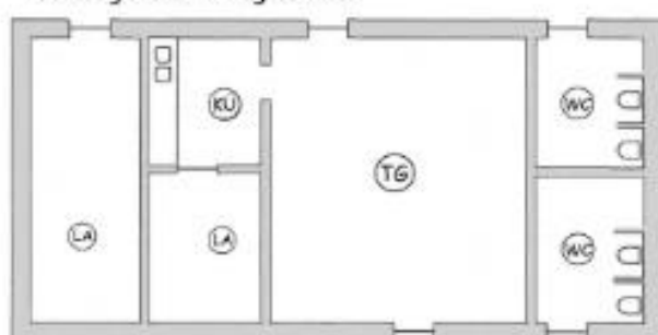
Nebengebäude Erdgeschoss
