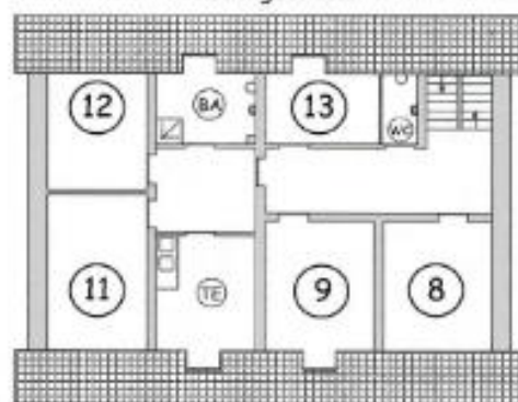
Dachgeschoss
